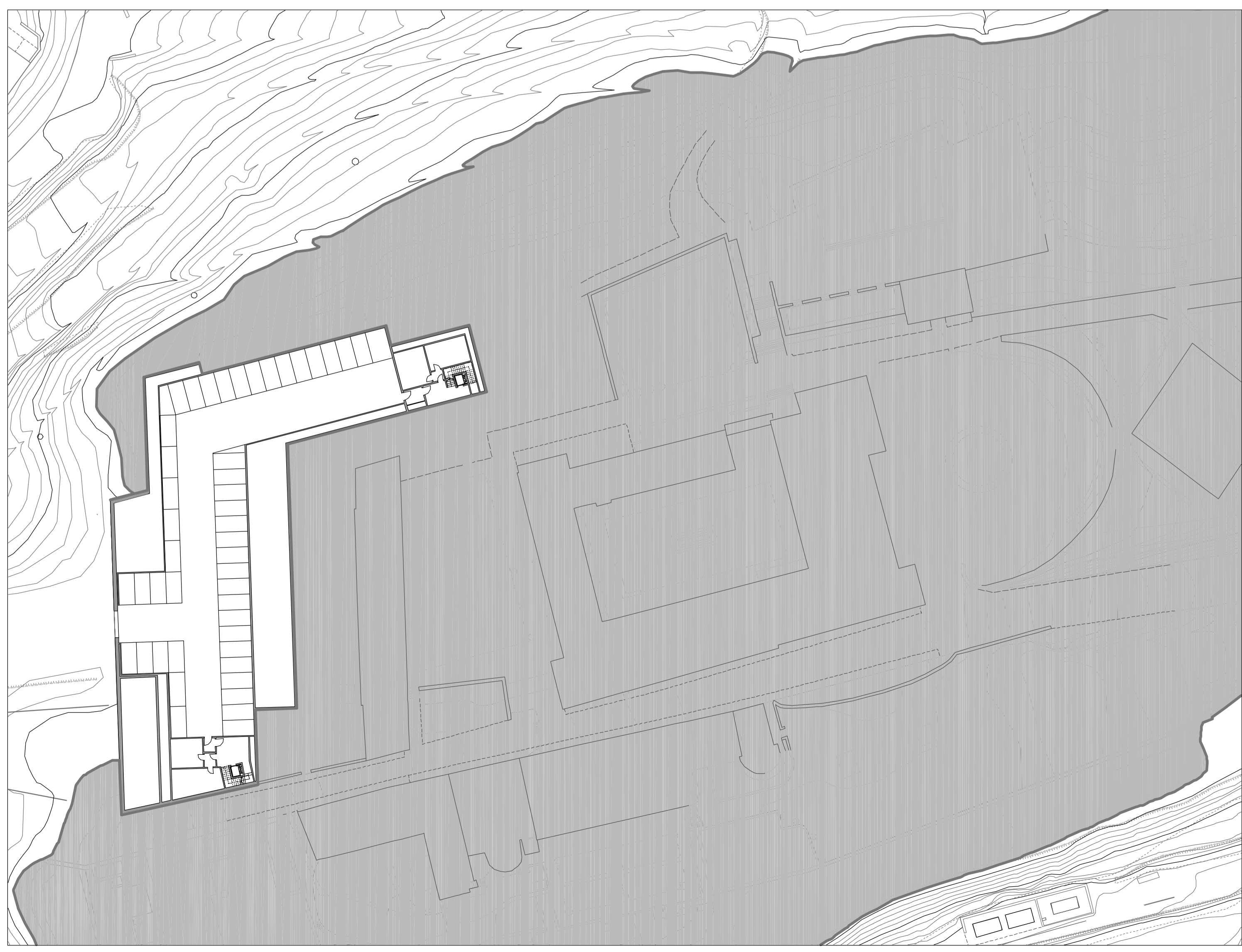
PLANIMETRIA GENERALE LIVELLO 3 - 328,5m
